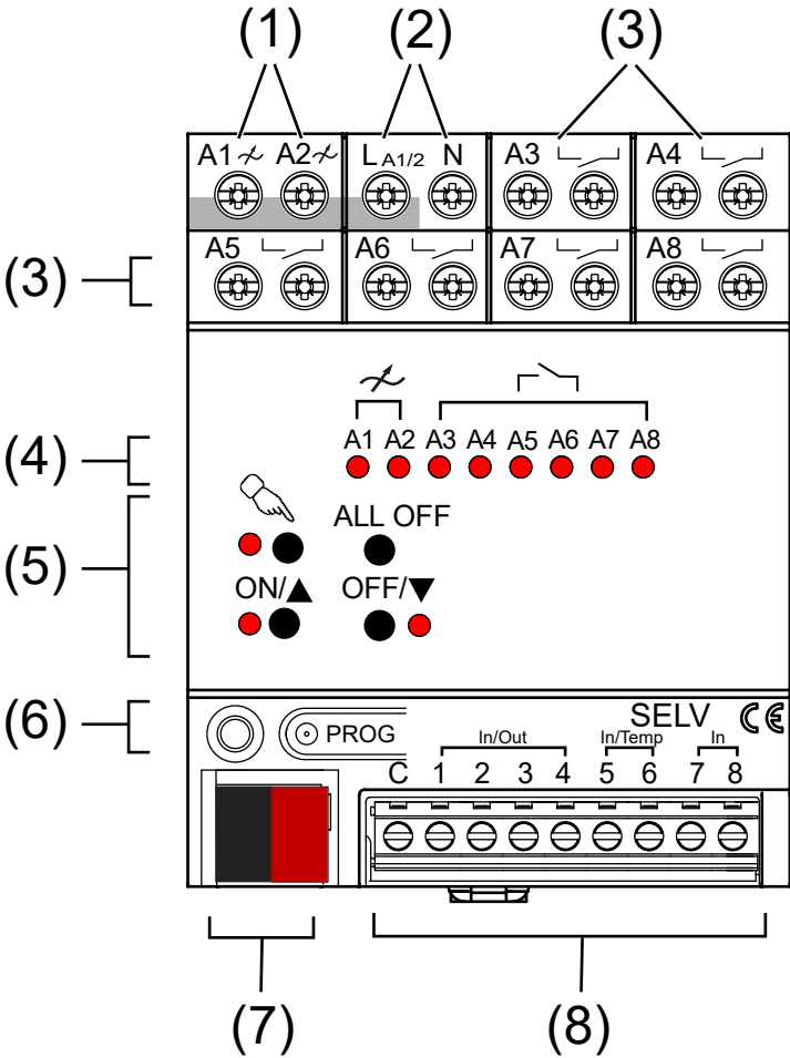
Figure 1: Vue de face de l'appareil
