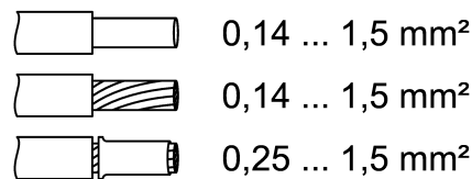
Figure 10: Section de conducteur serrable, postes auxiliaires
