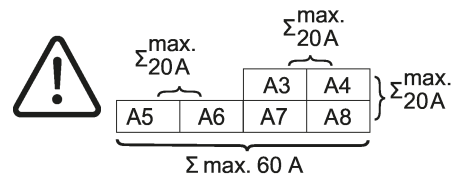
Figure 7: Intensité maximale admissible des sorties voisines
