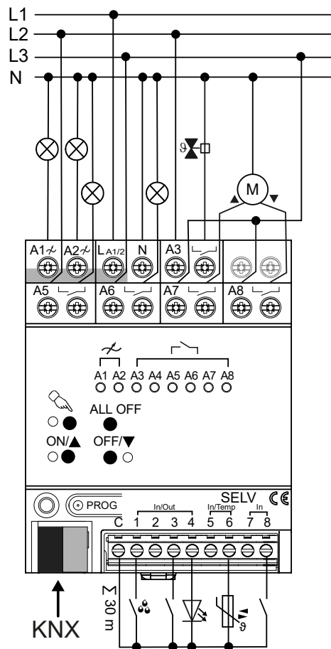
Figure 5: Exemple de raccordement de charges en général
