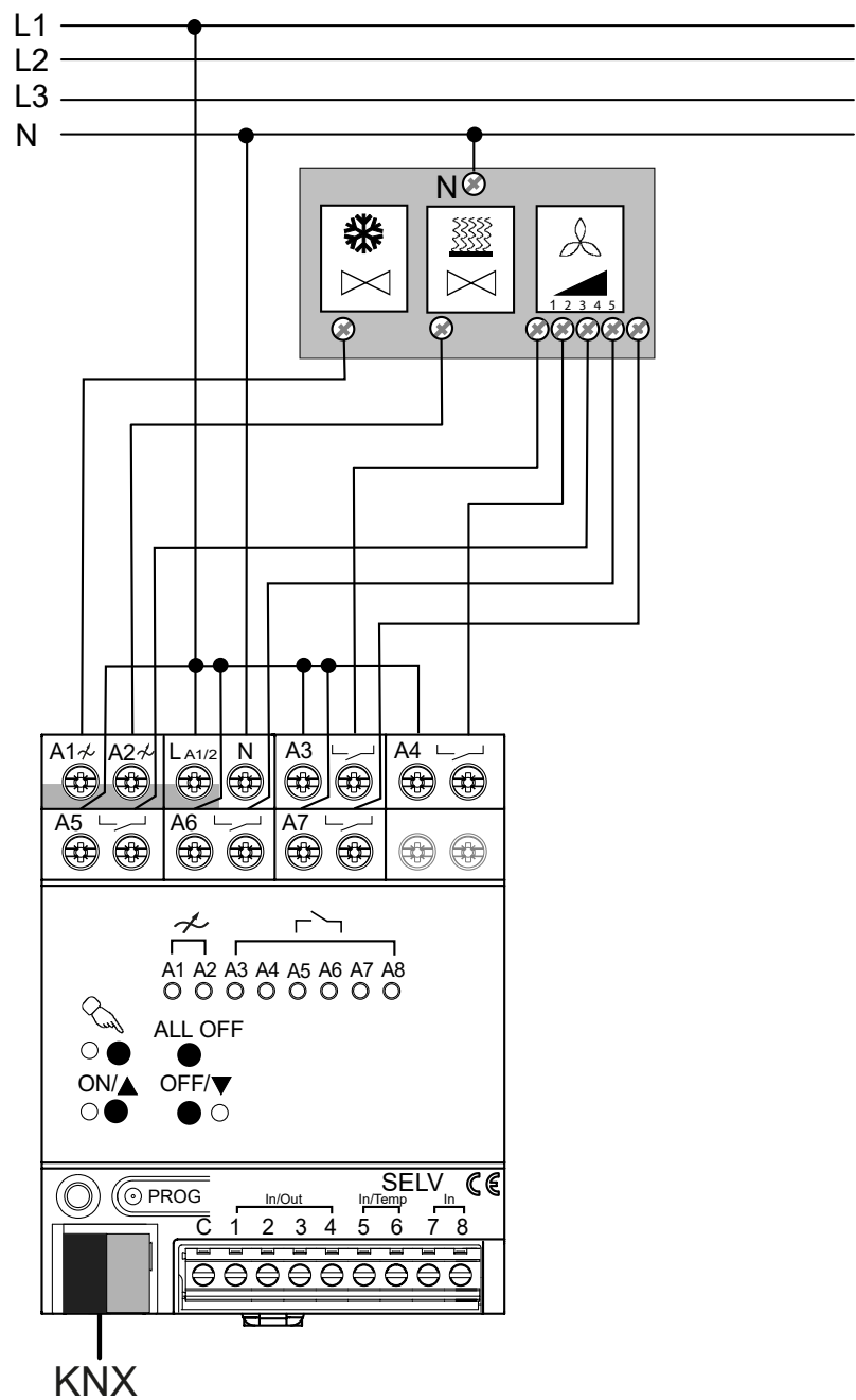
Figure 3: Exemple de raccordement pour 1 ventilo-convecteur via des sorties de variation et des sorties relais
