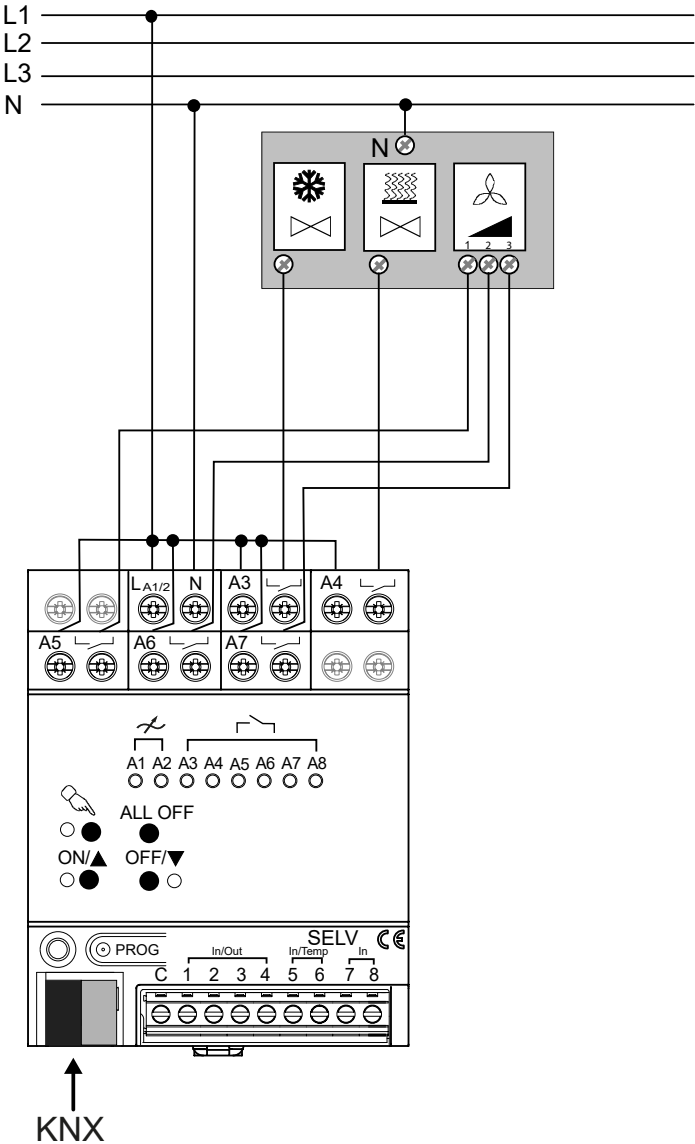
Figure 4: Exemple de raccordement pour 1 ventilo-convecteur via des sorties relais
