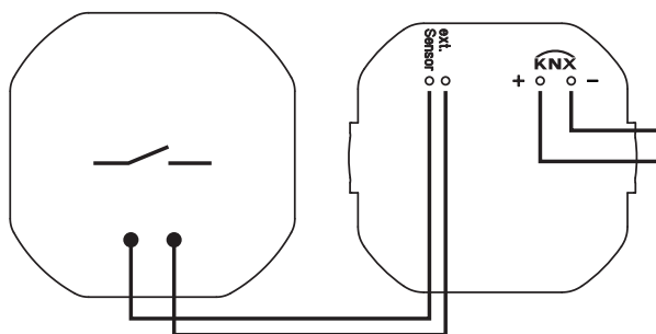
Fig. 3: Raccordement de l'appareil
