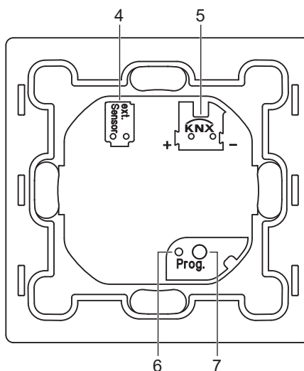
Fig. 2: Conception de l'appareil
