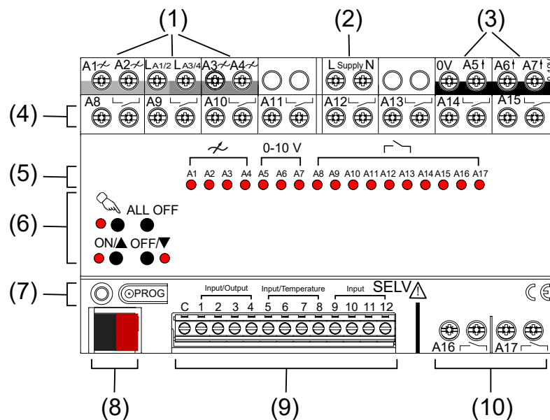
Bild 1: Geräteaufbau Frontansicht
