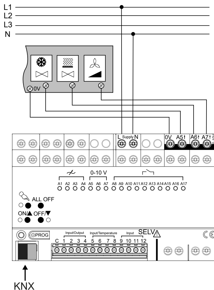
Bild 4: Anschlussbeispiel für 1 FanCoil über Analogausgänge 0-10V
