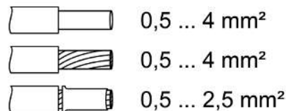
Bild 10: Klemmbare Leiterquerschnitte Lastausgänge und Spannungsversorgung
