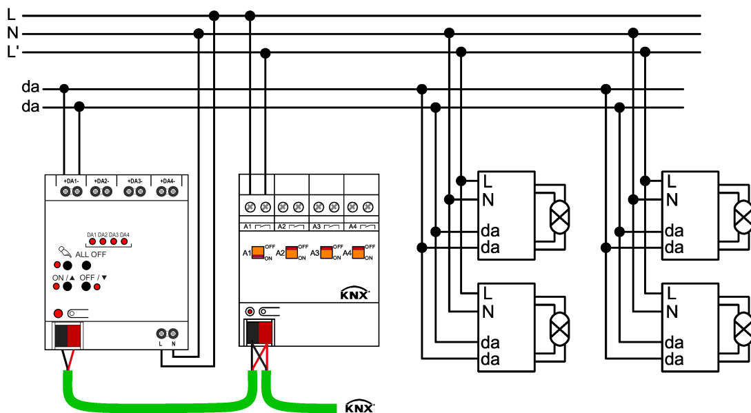
Bild 9: Beispiel eines Anschluss-Schemas zur Standby-Abschaltung durch einen KNX Schaltaktor
