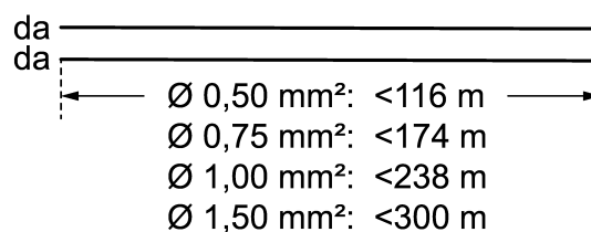
Bild 2: Leitungslänge DALI
