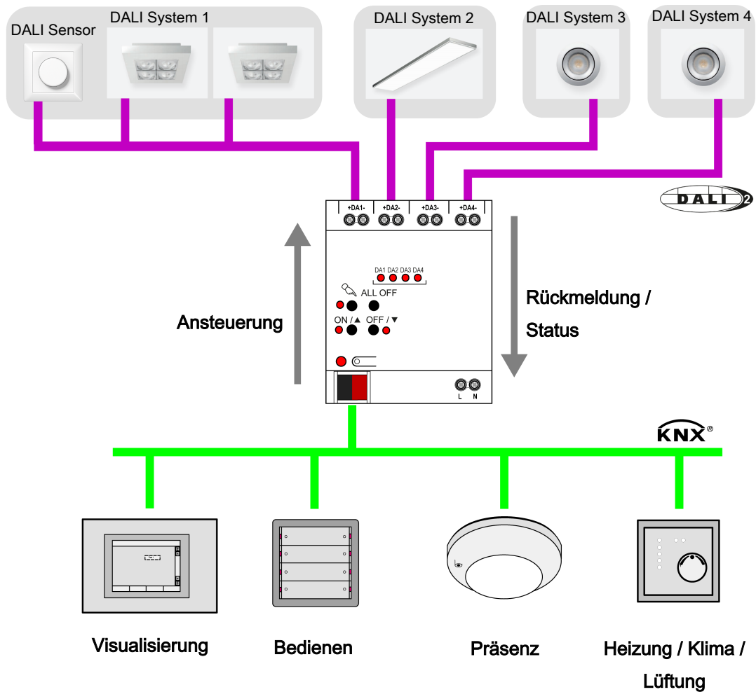
Bild 5: Prinzipübersicht einer KNX DALI Systemanbindung (Beispiel)
