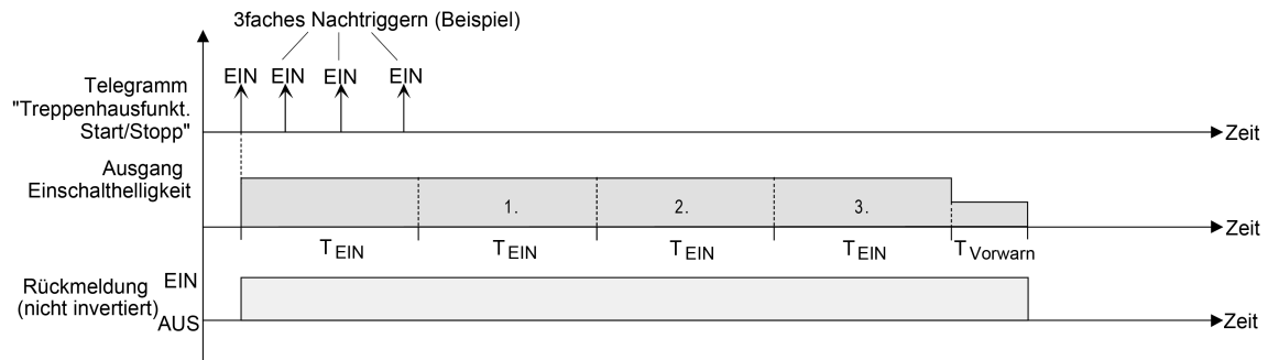
Bild 44: Zeitverlängerung der Treppenhausfunktion
