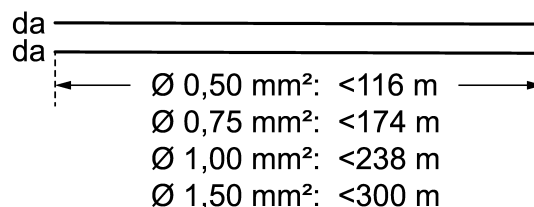
Bild 3: Leitungslänge DALI
