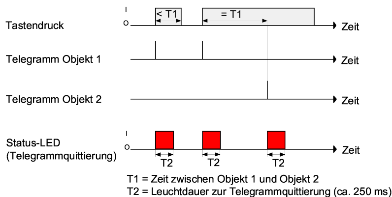
Bild 25: Beispiel zum Bedienkonzept "Objekt 1 und Objekt 2"
