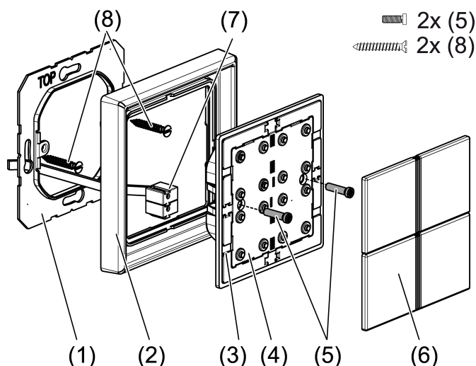
Bild 1: Montage Tastsensor-Modul
